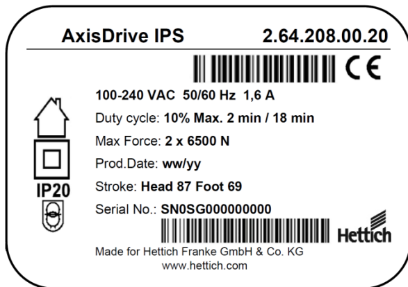
Abb. 4: Typenschild
