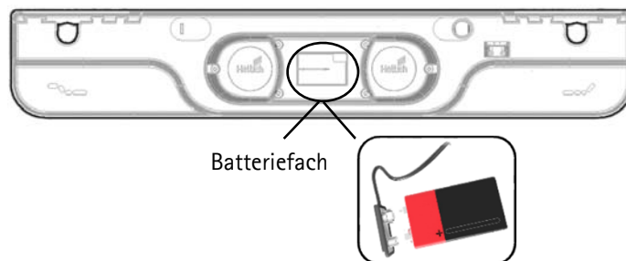
Abb. 16: Blockbatterie
